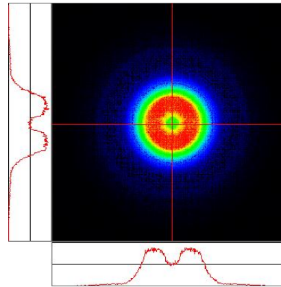
放射照度分布
