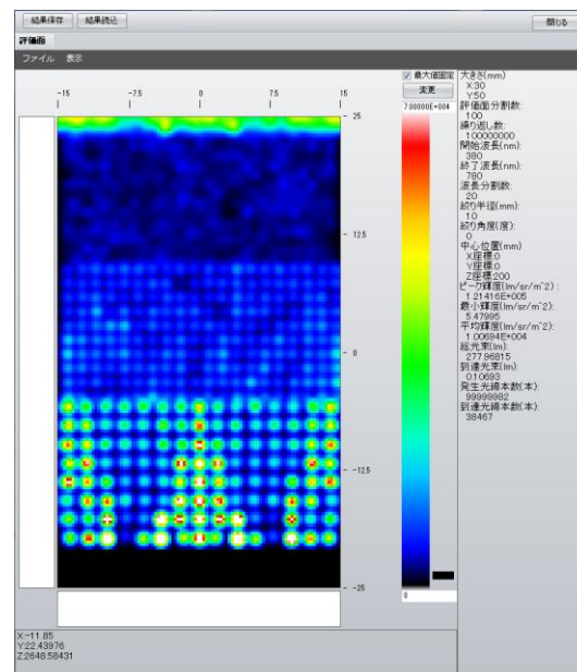
輝度分布
